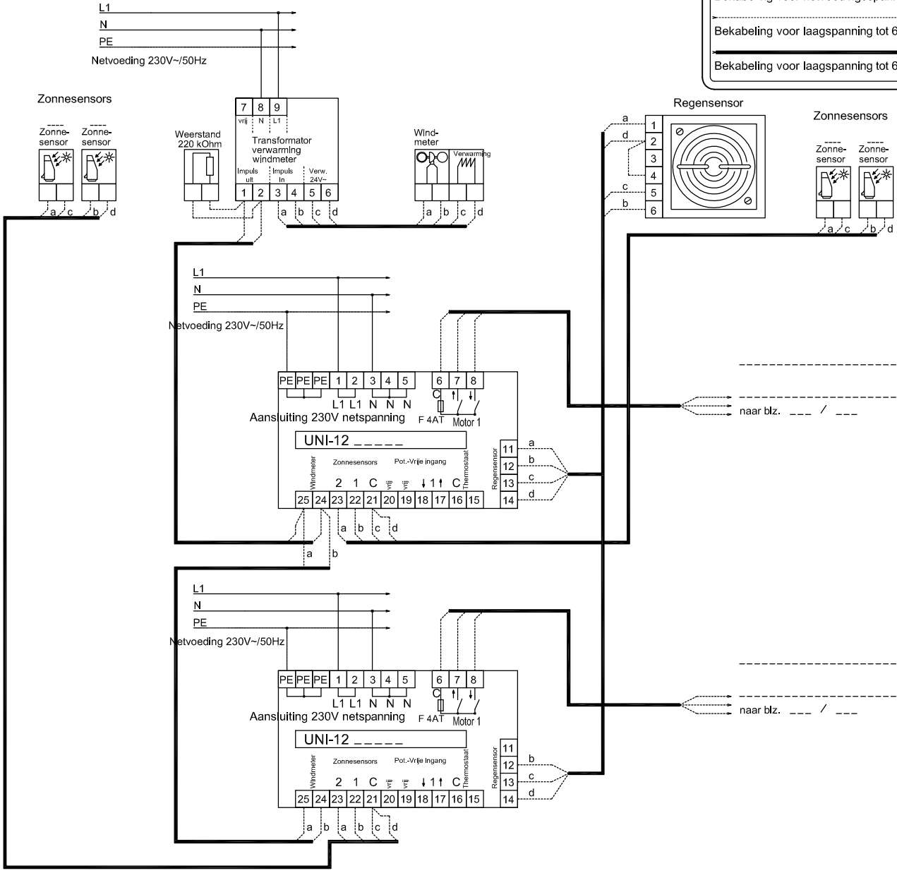
PRINCIPE AANSLUITSCHAMA UNI12 / UNI12 / Sensors
