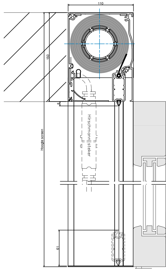
Doorsnede BB
